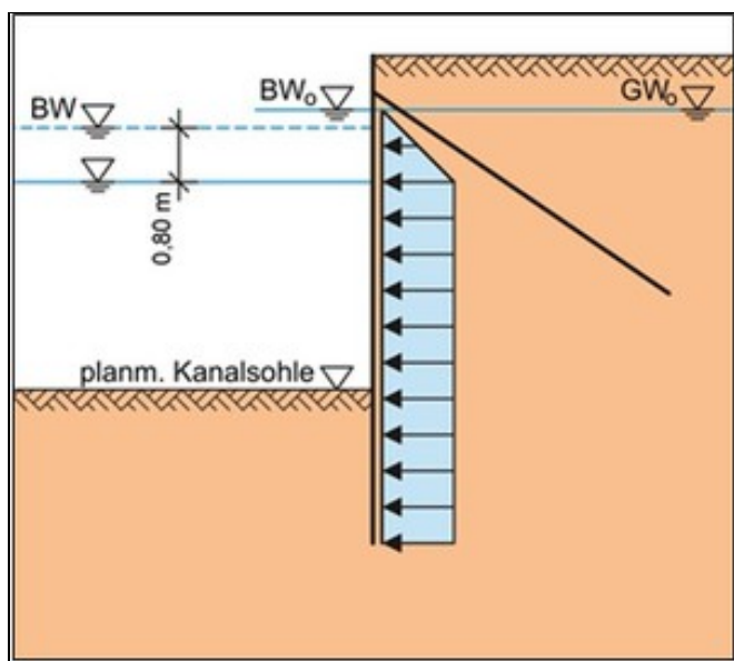
Bild 4: Wasserdruckansatz für Fall A, BS und P
