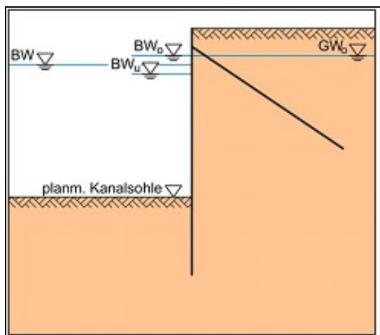
Bild 1: Hydraulische Randbedingung in Fall A
