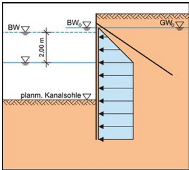
Bild 5: Wasserdruckansatz für Fall A, BS und A-1
