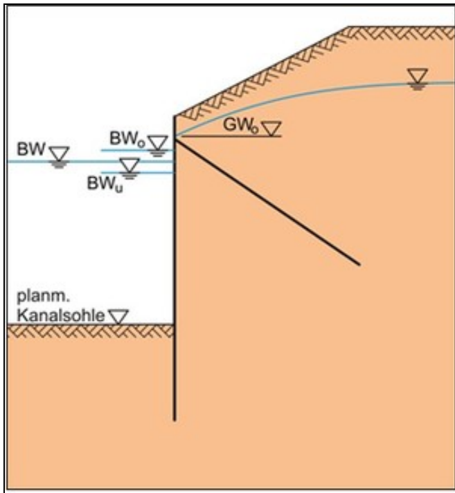
Bild 2: Hydraulische Randbedingungen in Fall B
