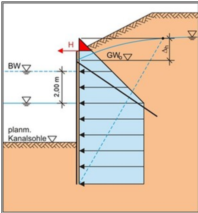
Bild 8: Wasserdruckansatz für Fall B, BS-A 1
